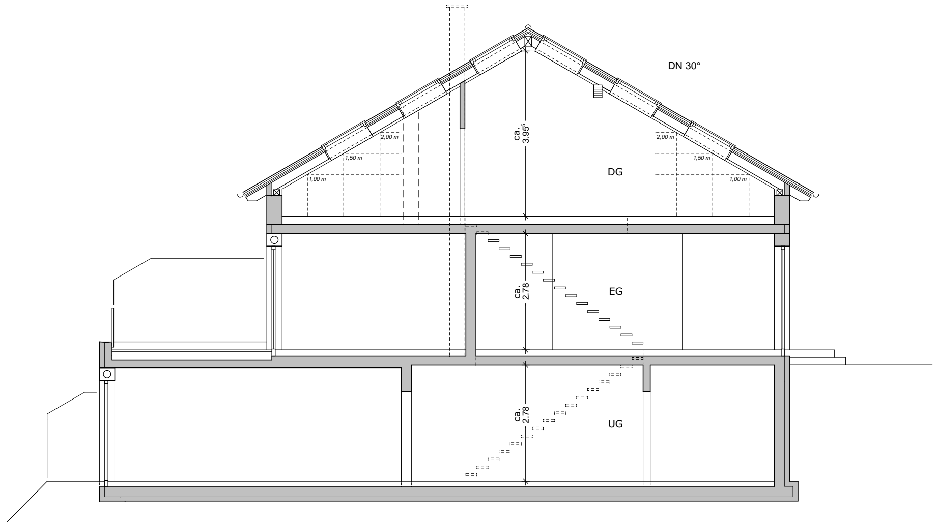
DHH 2 - Schnitt
