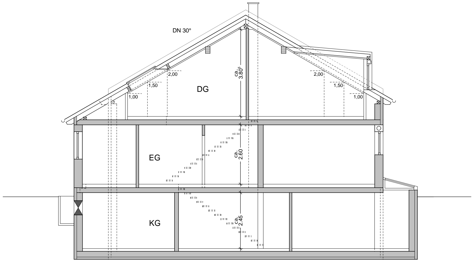
DHH 1 - Schnitt
