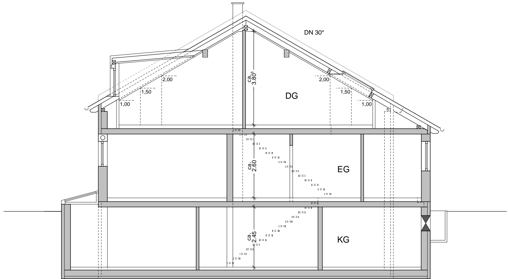
DHH 2 - Schnitt
